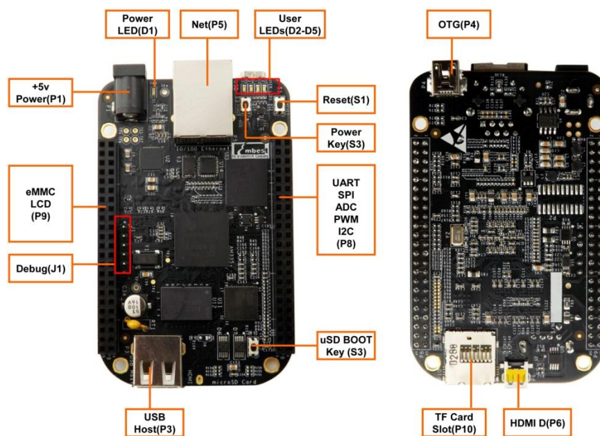
图 2-4 接口/按钮/LED
